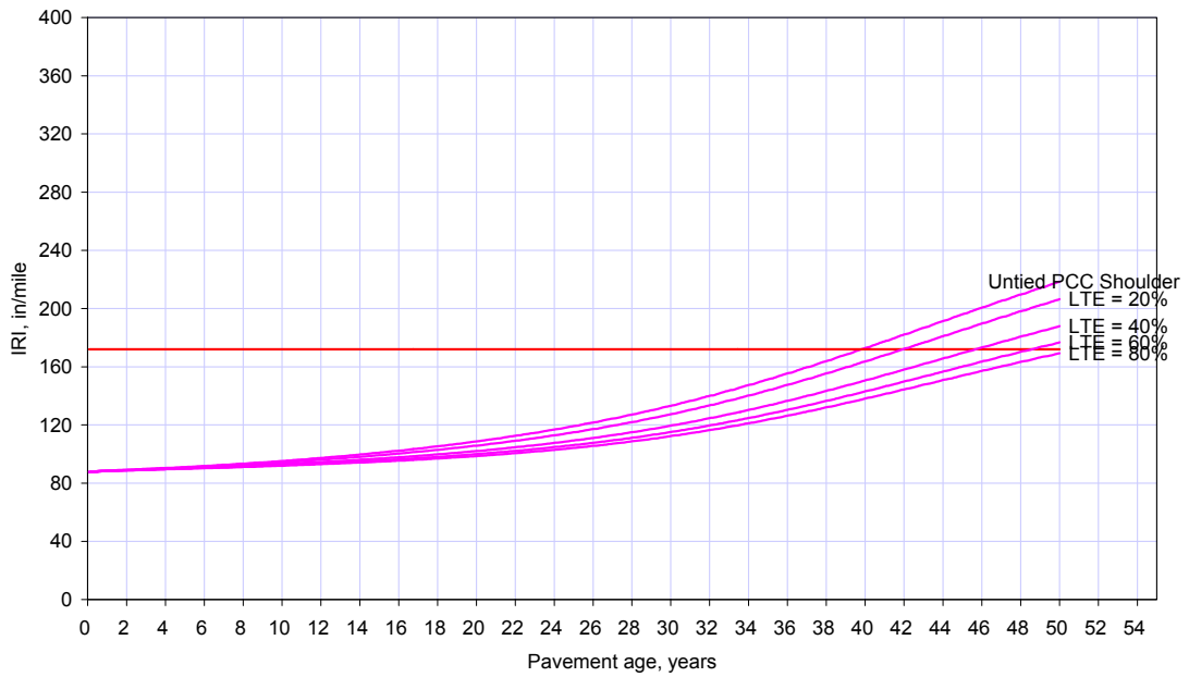
Predicted IRI
