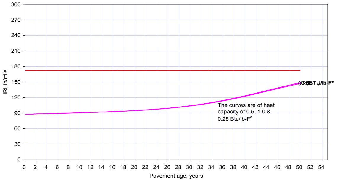
Predicted IRI
